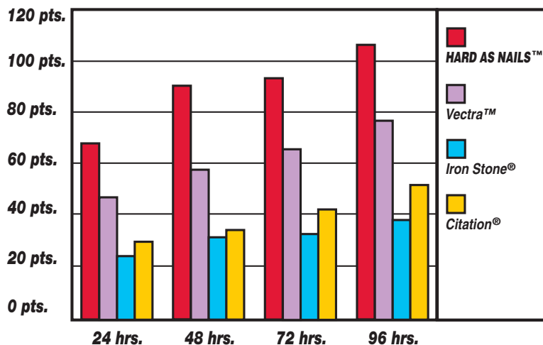
*Koenig Pendulum Hardness Tester
